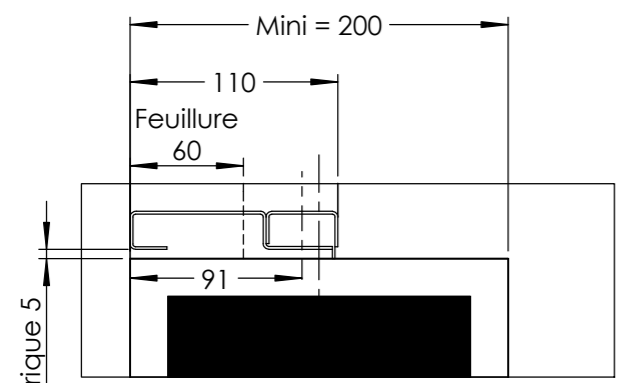
DÉTAIL A
